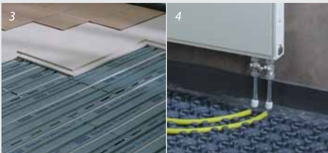
3 Ενδοδαπέδια θέρμανση με το σύστημα ROTEX secco. Σύστημα ξηρής εγκατάστασης με τσιμεντοσανίδες
